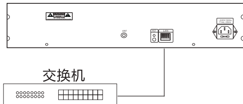
基本连接图
