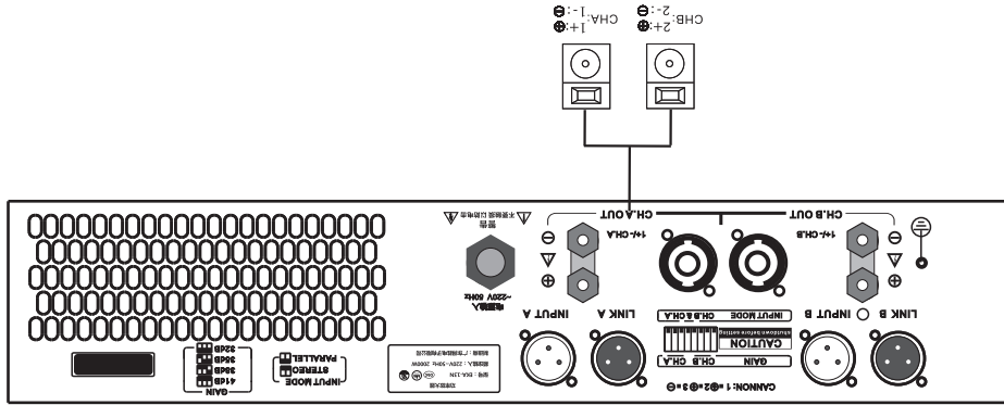
Wiring method 2 :
